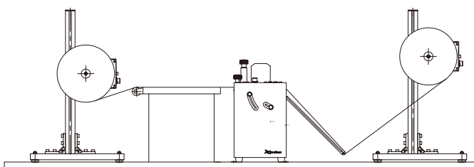
ZKF-25との組合せによるシート検査
