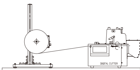
ZKC-25との組合せによるフィルム切断
